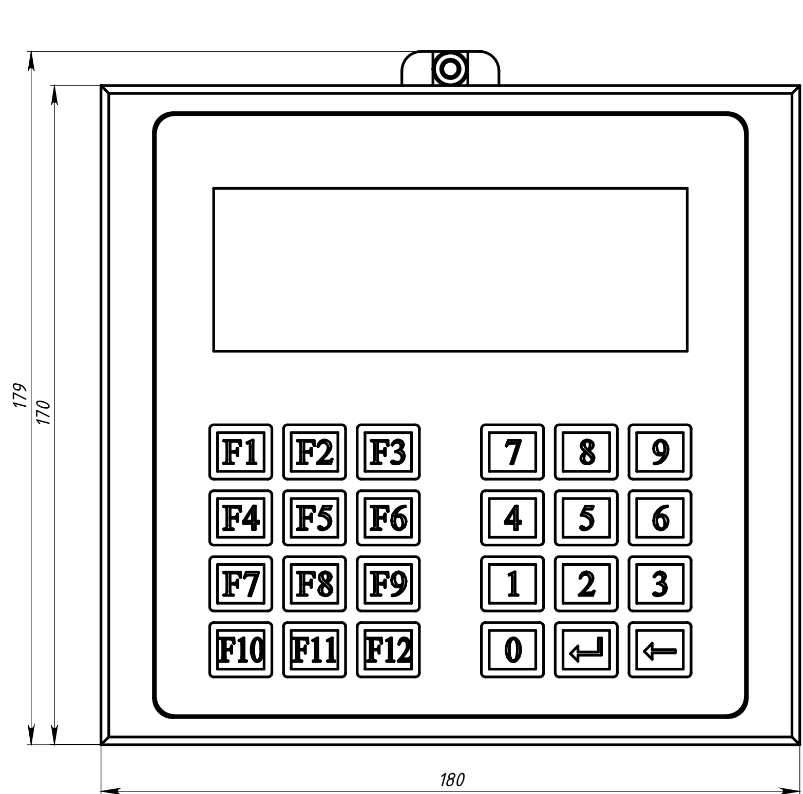
Установочные размеры для монтажа (1 : 2)
