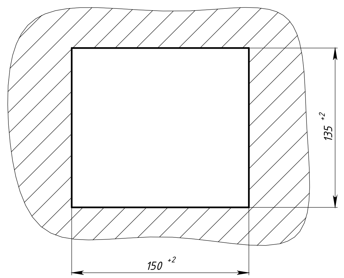
Установочные размеры для монтажа (1 : 2)
